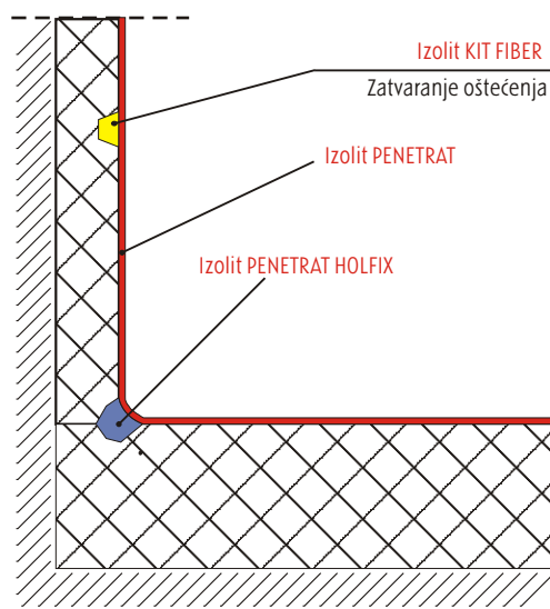
Detalj A
